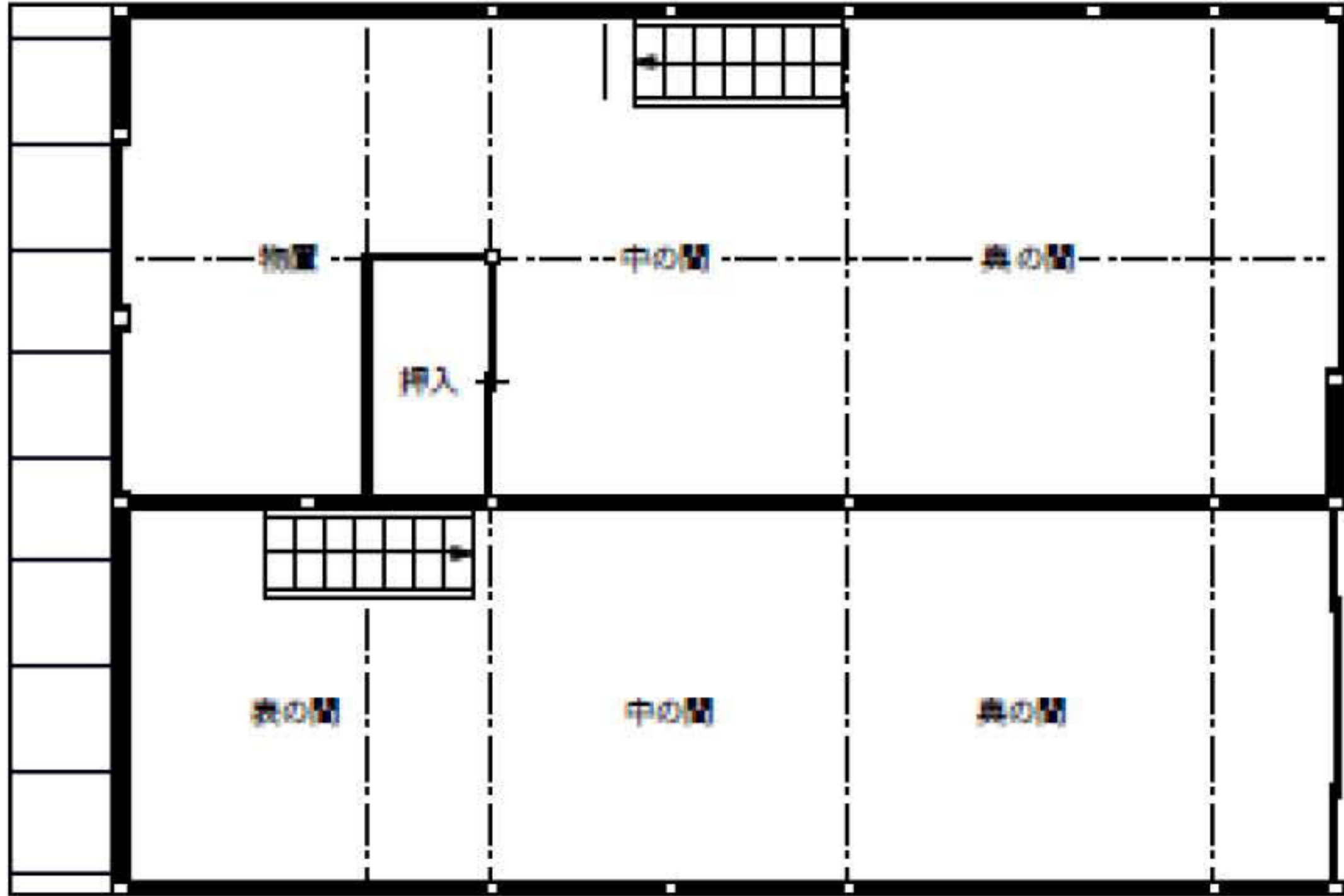
2階 PLAN
