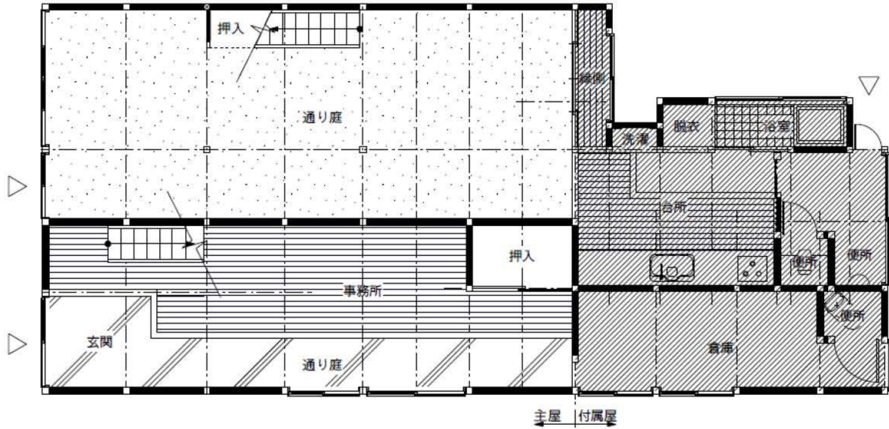
1階 PLAN
